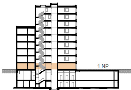
ŘEZ
